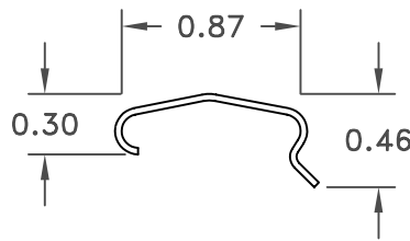
F Cleat (Metal)
