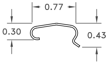
C Cleat (Metal)
